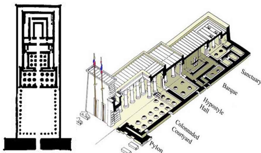
شکل 7 نمای پلان معابد مصری در ادفو
