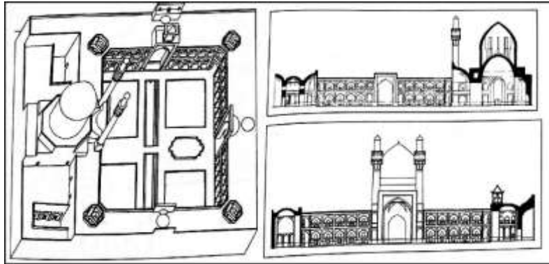
پلان ۲: نما، برش و سه بعدی از مدرسه چهارباغ اصفهان (پیرنیا، ۱۳۸۷، ص. ۳۳۴)
