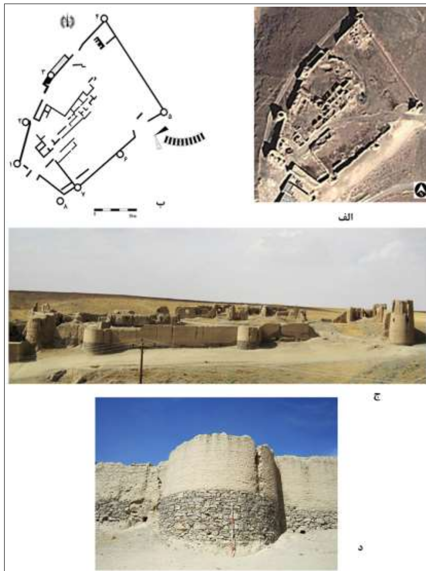
تصویر ۳: تصویر هوایی، نقشه، نمای ضلع جنوب شرقی و برج شماره ۷ قلعه لک (نگارندگان، ۱۳۹۲)
