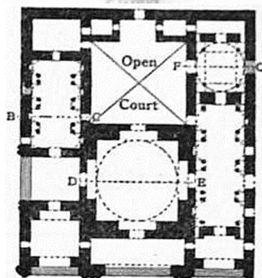
شکل 11 پلان و برش عمودی کاخ سروستان (پوپ، 1385: 63)
