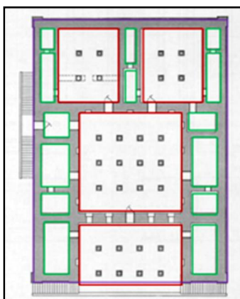
پلان 6 جزئیات فضاهای کاخ خشایار شاه
