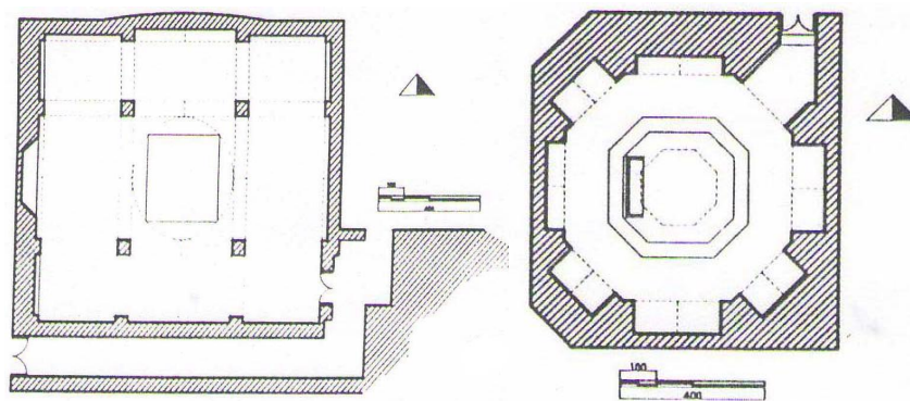
شکل ۱۱ الف. پلان کنیسه ملایعقوب؛ ب. پلان کنیسه حاجی الیاهو در جوباره
